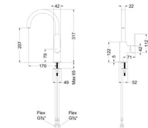
Wastafelmengkraan draaibare uitloop - Forma
