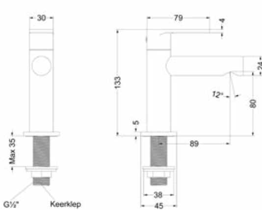
Fonteinkraan staand model S - Forma
