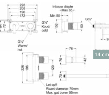
Inbouw wastafelkraan incl. inbouwbox - Stilo
