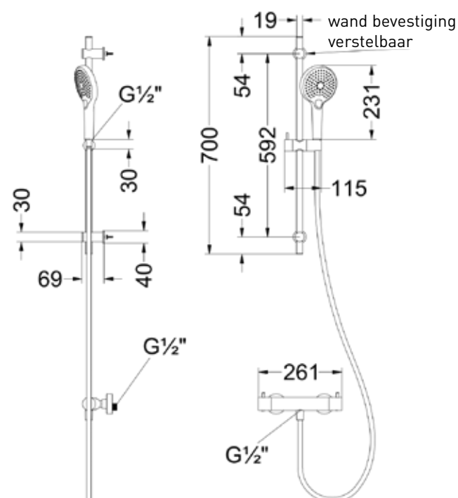
Douchethermostaat opbouw
