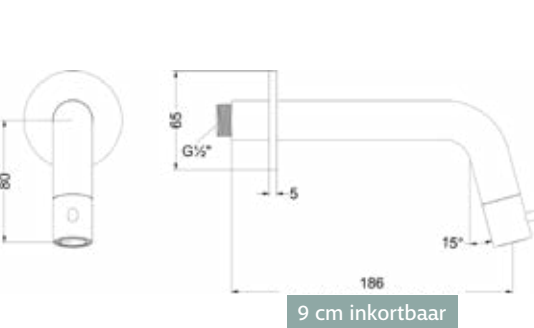
Fonteinkraan wandmodel inkortbaar - Stilo
