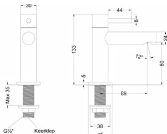
Fonteinkraan staand model S - Stilo
