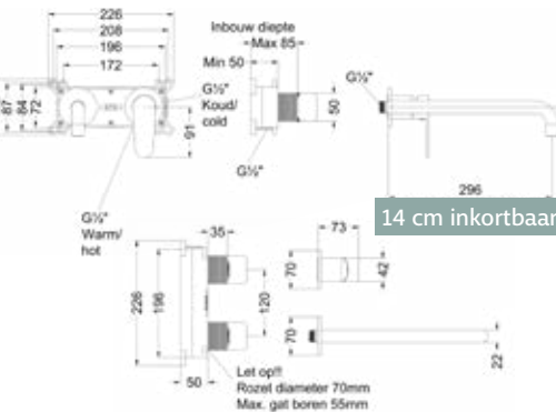
Inbouw wastafelkraan incl. inbouwbox - Forma
